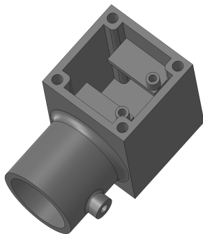
Obr. 9: Model senzorového modulu
