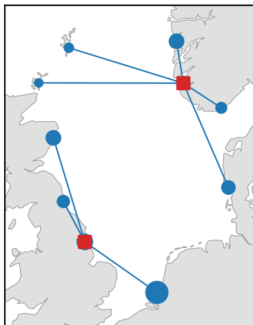
(d) p -center, p = 2
