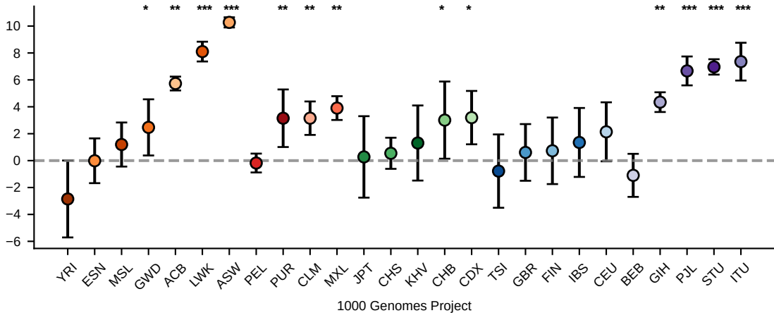
Cophylogeny score
