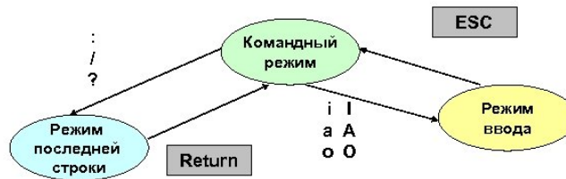
Рисунок 6.1: Граф
