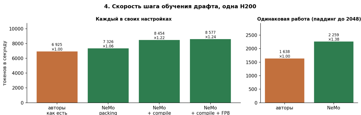
Рис. 3: Скорость шага обучения драфта на одной H200.
