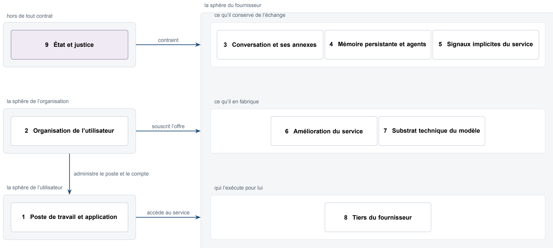
Figure 1 – Chaque maillon est situé par la sphère qui le maîtrise et, chez le fournisseur, par la fonction qu'il y remplit. Les liens sont des rapports d'autorité ou de contrat, non des circulations d'information.
