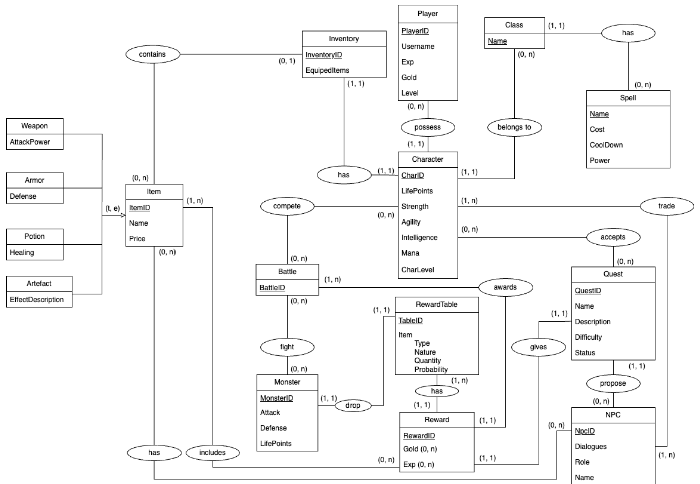
Figure 1: Diagramme Entité-Association du système
