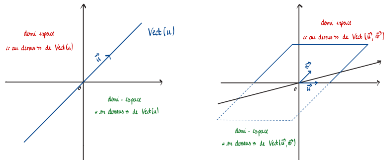
FIGURE 1 – Intuitivement, en dimension finie, un hyperplan peut être vu comme une « tranche » de l'espace ambiant, le séparant en deux parties.
