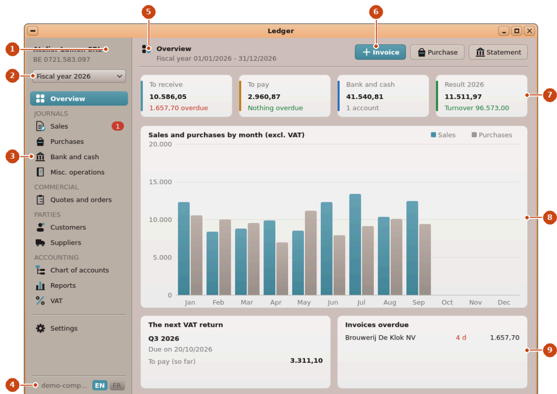
La page Overview (vue d'ensemble) de la société de démonstration, et les parties de la fenêtre.
