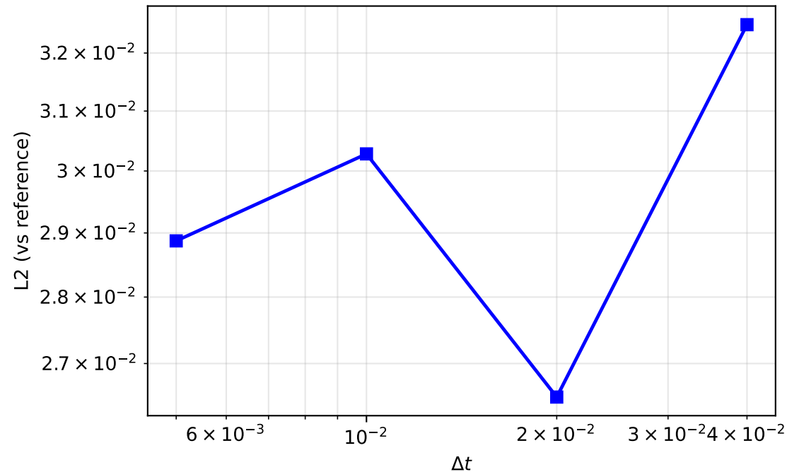
FHN: L2 vs dt (N=2000)
