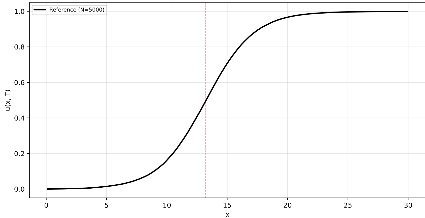
FHN: profiles ( T=5.0 , a=0.25 , \nu=0.5 )
