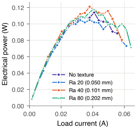
Fan 700 rpm (14.5 m/s)
