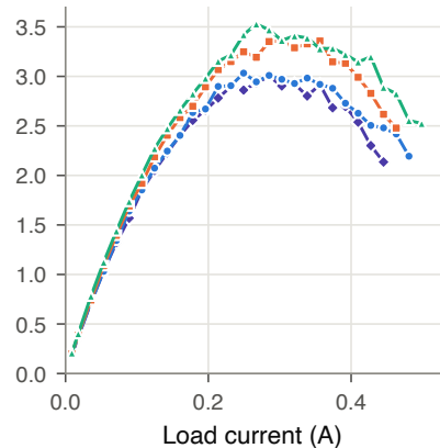
Fan 1700 rpm (35.8 m/s)
