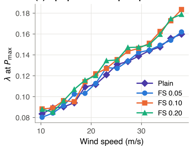
(d) Tip-speed ratio at peak power
