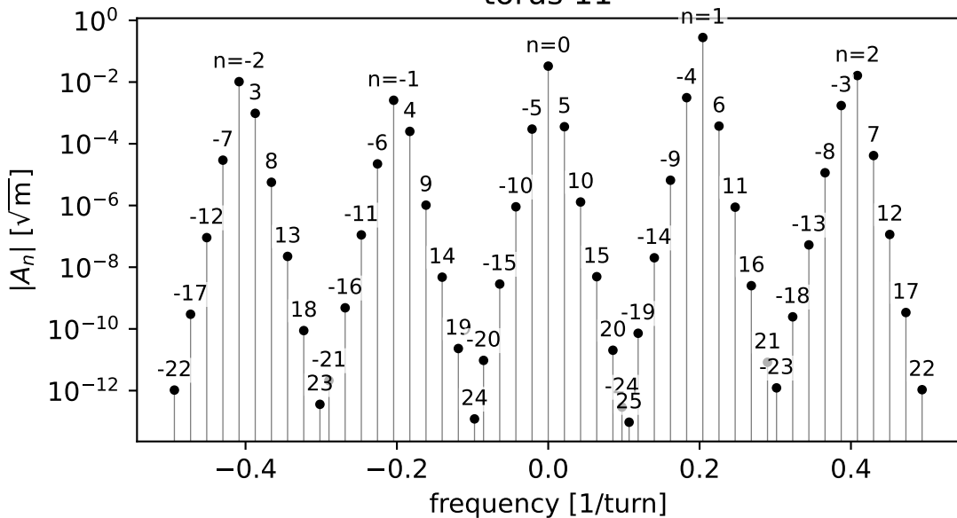
torus 11
