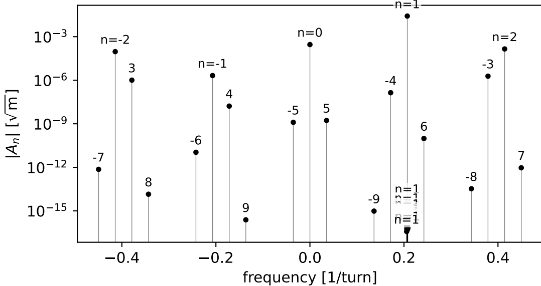
torus 1
