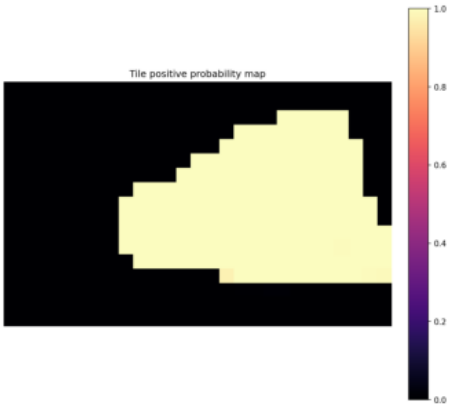
tile_prob_map.png
