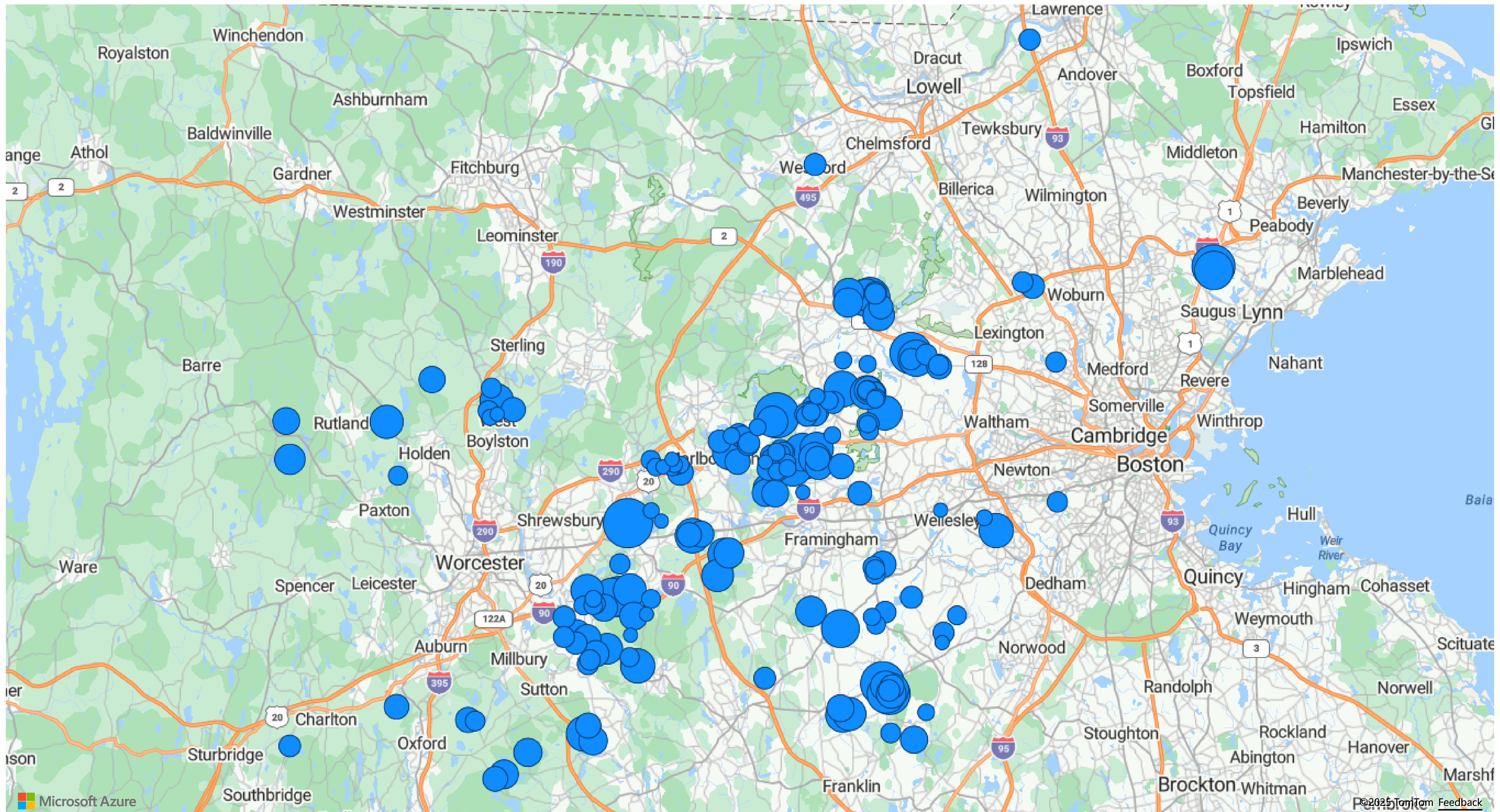
Conteggio di reviews per latitude e longitude
