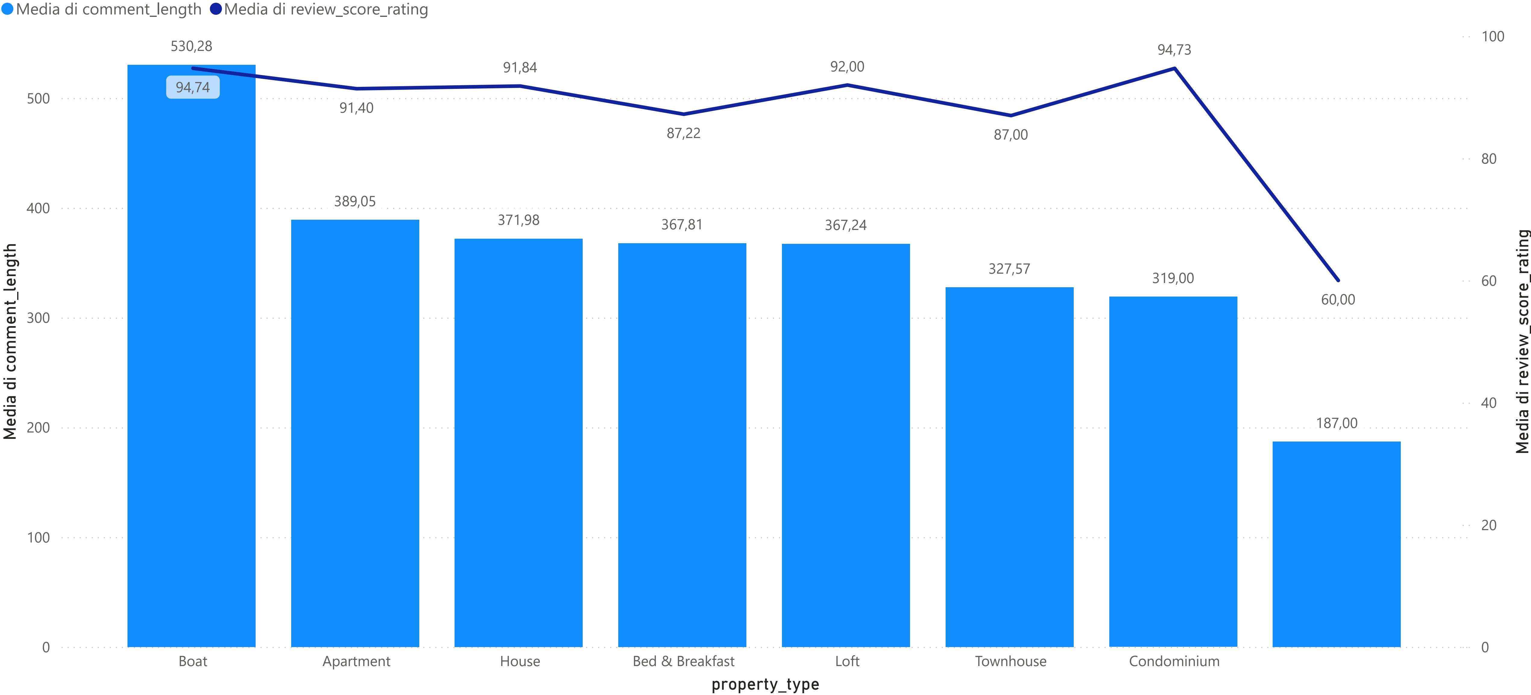
Media di comment_length e media di review_score_rating per property_type
