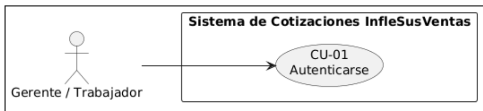
Figura 10. CU-01 Autenticarse
