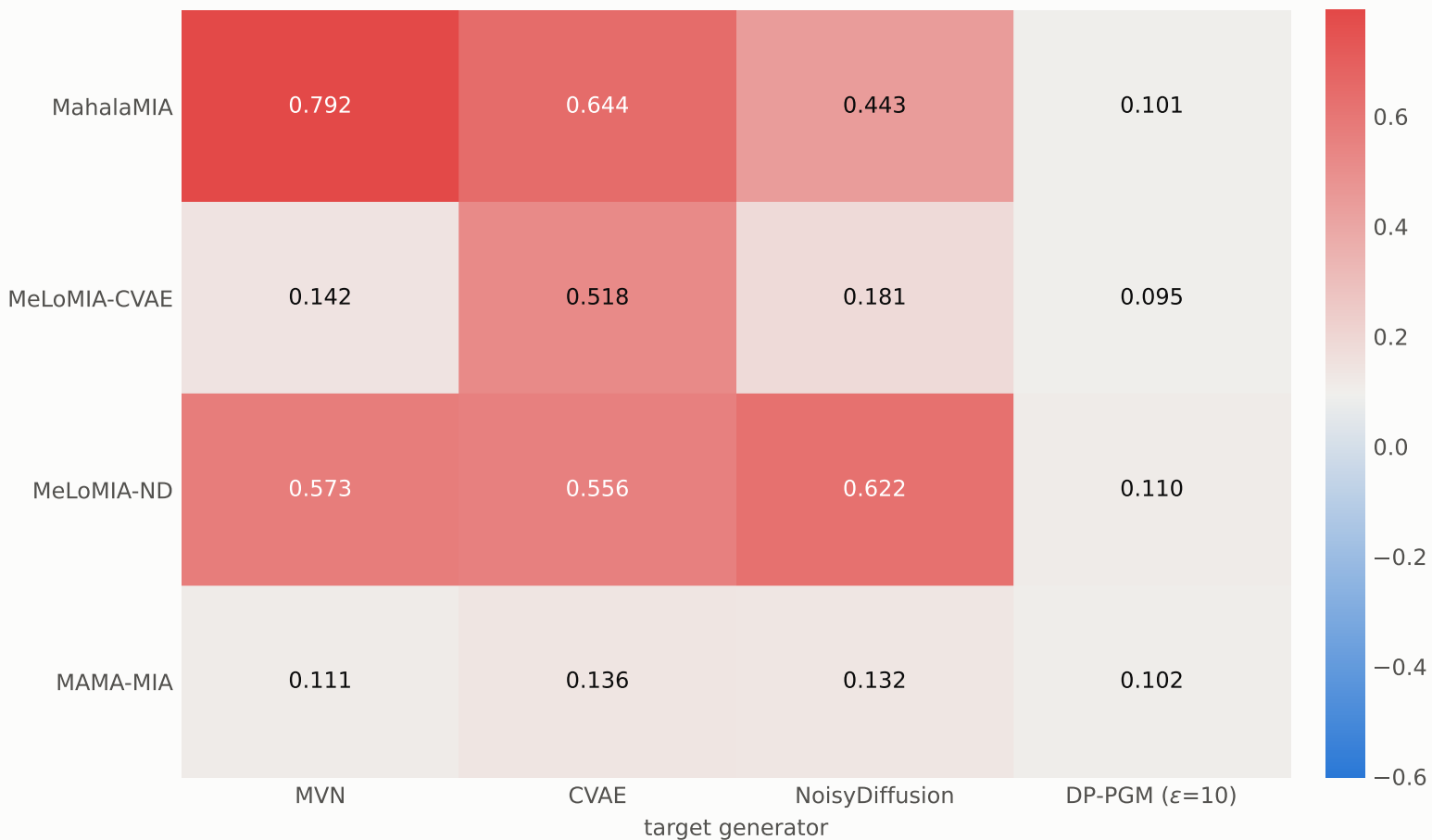
TPR @ 10% FPR — BRCA
