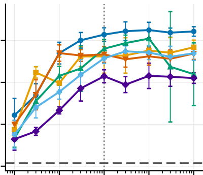
CoBP-RA
