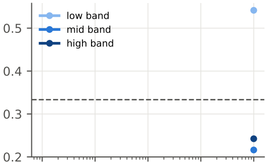
PrivBayes · DCR
