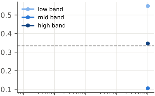
PrivBayes · DCR
