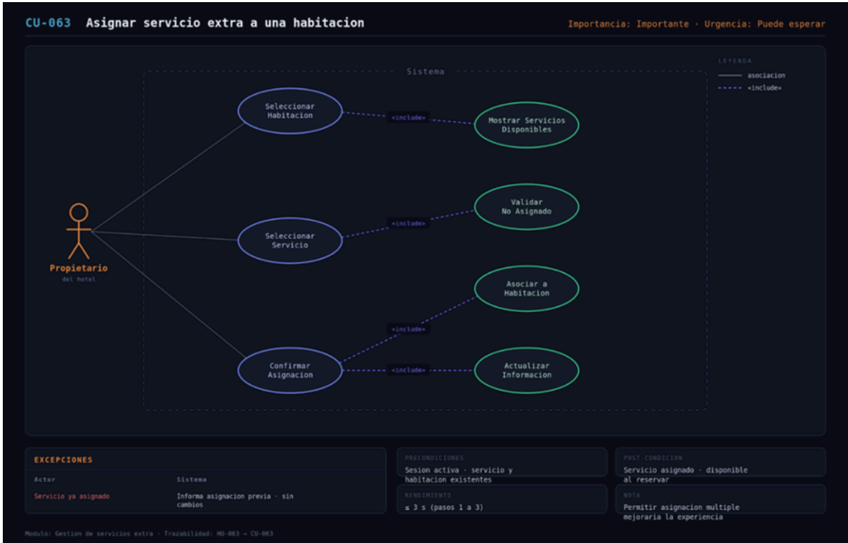
Diagrama UML de casos de uso
