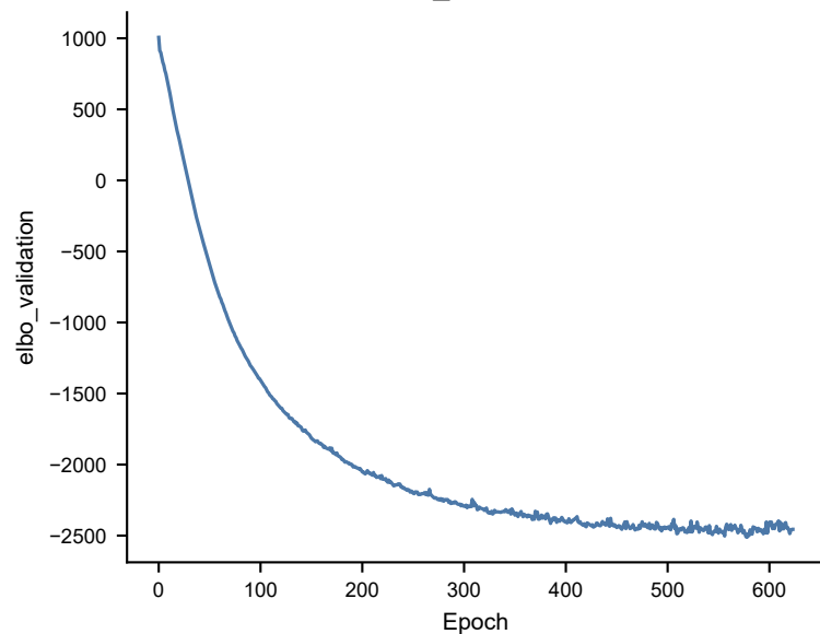
elbo_validation
