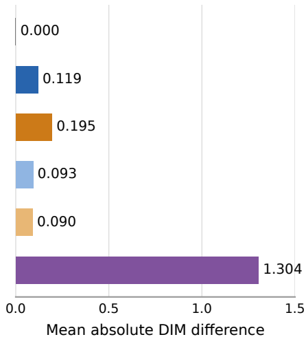
Llama 3.1 8B Instruct
