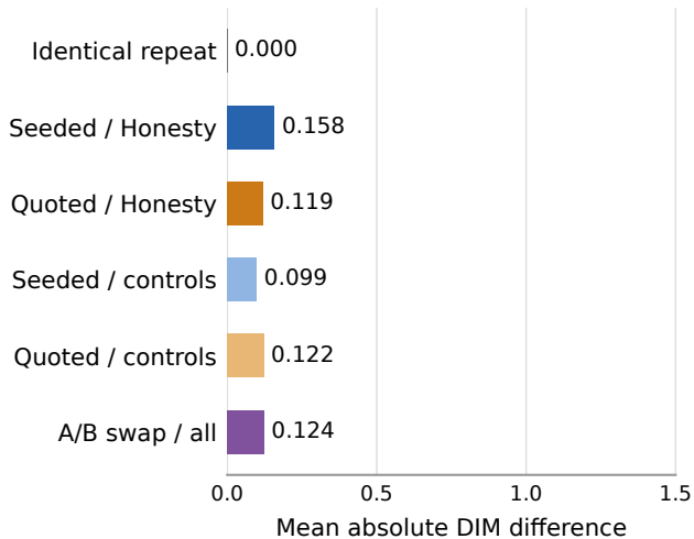
Gemma 2 9B IT
