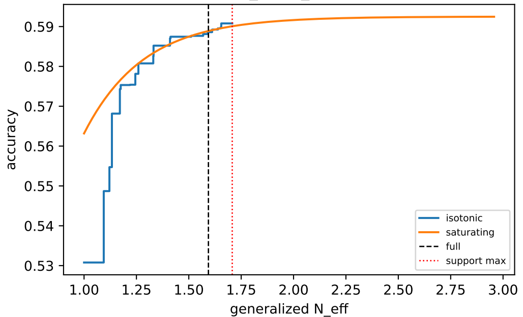
mind2web/C_uni / majority
