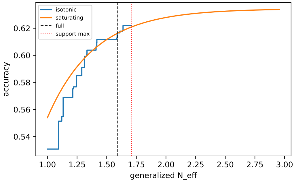
mind2web/C_uni / density
