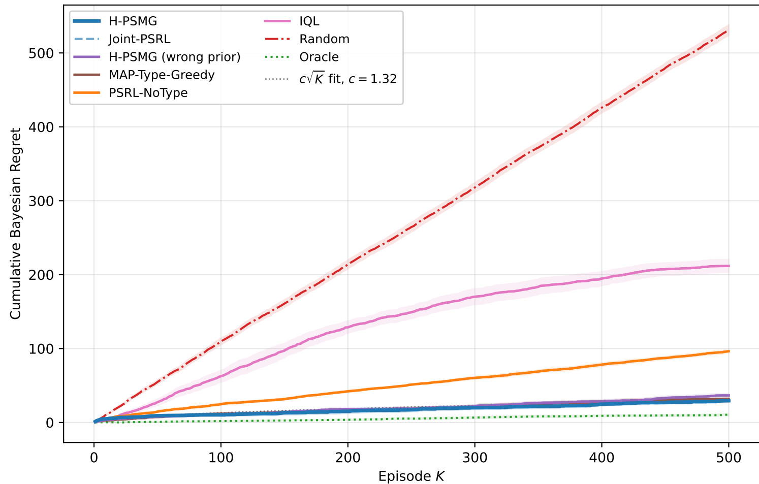
Cumulative regret on a 2-agent HT-MG ( S=3 , |\mathcal{A}_i|=2 , |\Theta_i|=2 , H=8 )
