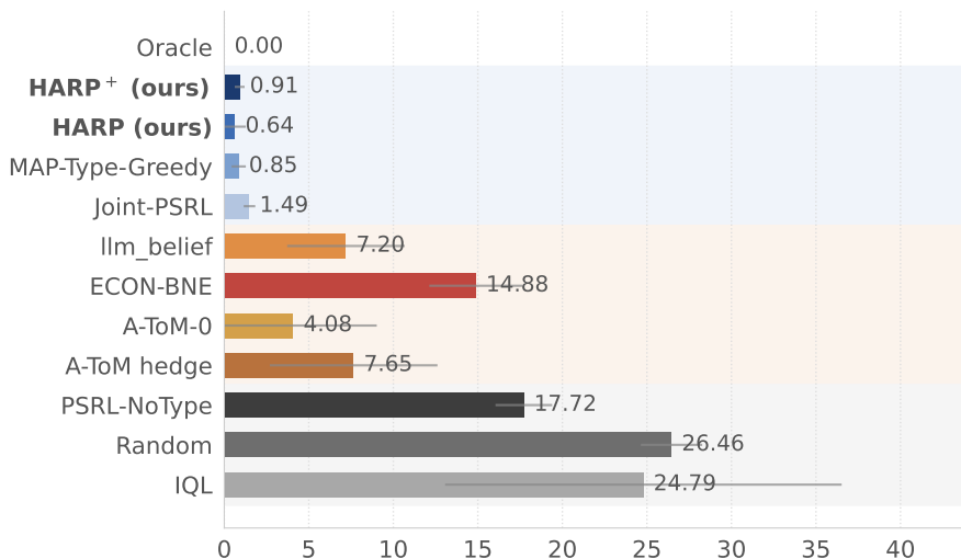
Llama-4-Maverick
