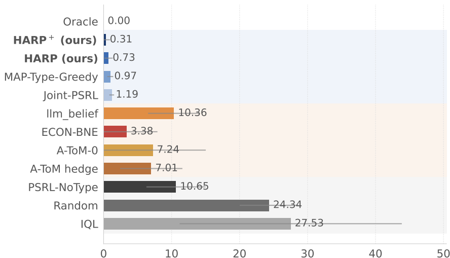
Llama-4-Maverick
