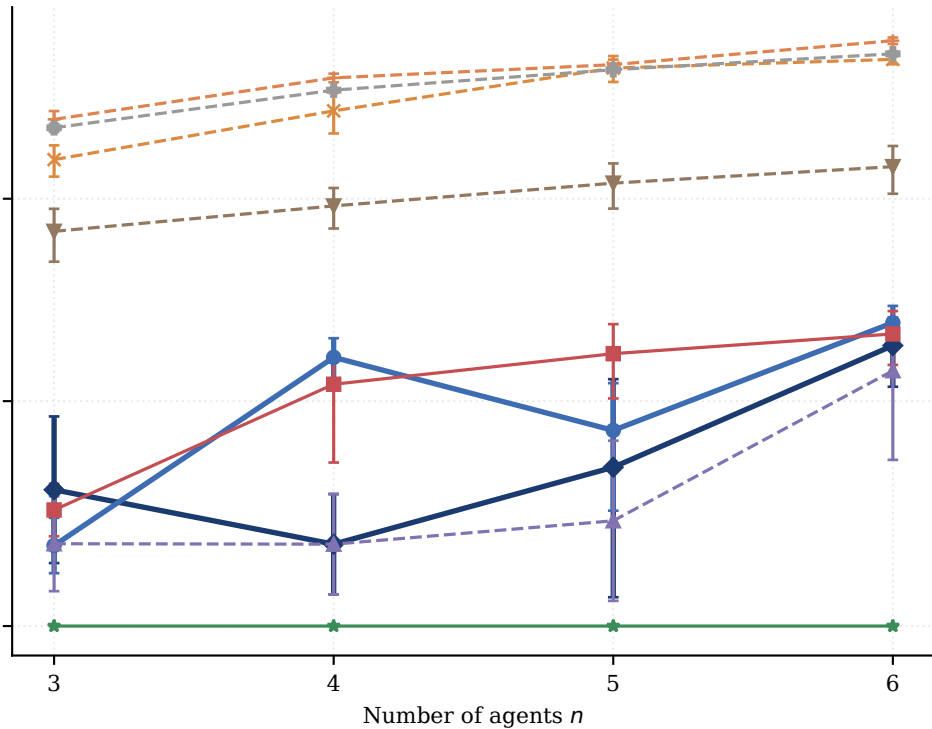
Llama-4-Maverick
