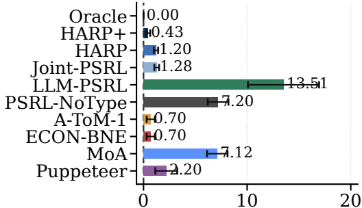
Llama-4-Maverick
