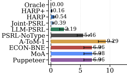
Llama-4-Maverick
