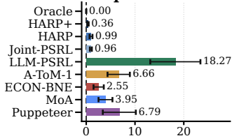
DeepSeek-V3.2
