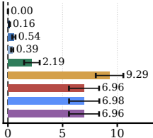
GPT-5.4-nano
