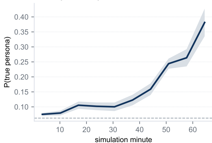
Exact persona posterior
