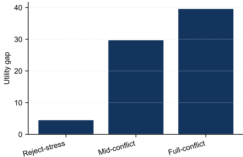
LLM-PACT minus best prompt
