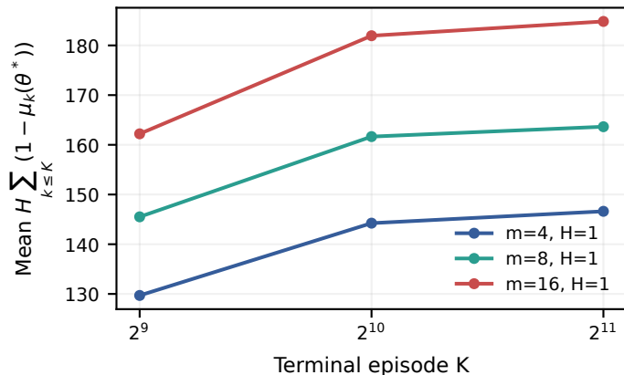
(d) K-independent type-error proxy
