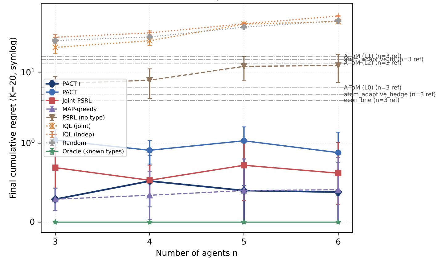
E-1.1 LLM tier: Kimi-K2.6
