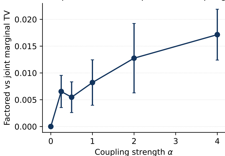
DeepSeek-V3.2-live: posterior coupling
