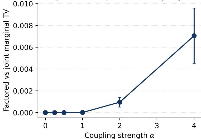
analytic-mixed: posterior coupling
