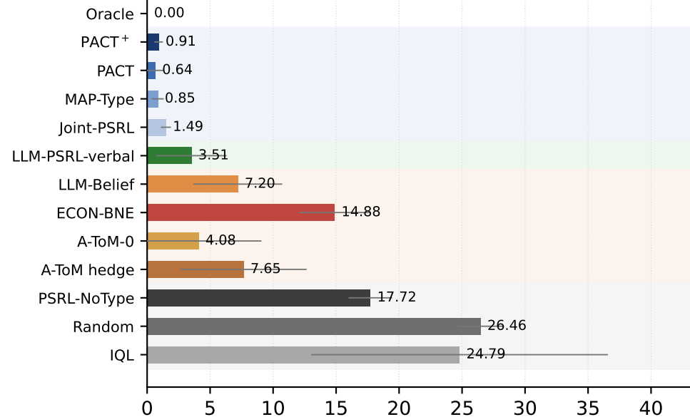
Llama-Maverick
