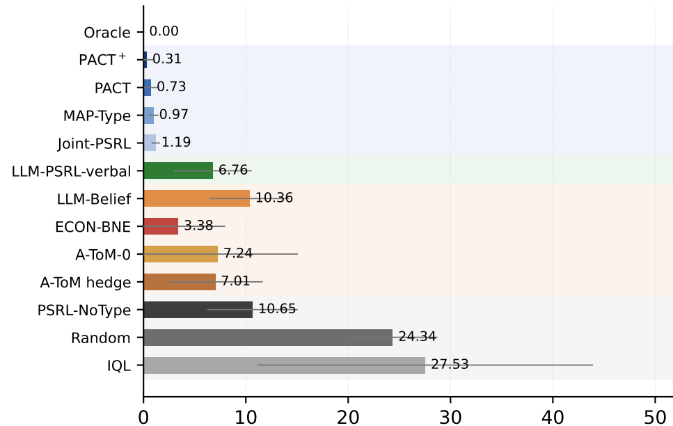
Llama-Maverick
