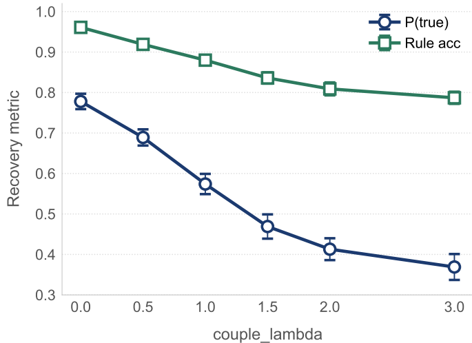
Posterior degrades
