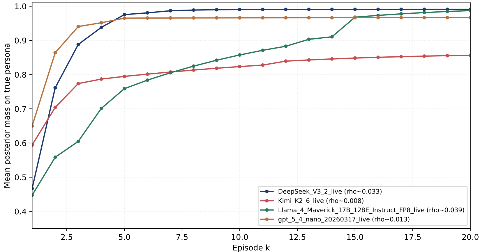
E-0.2 Posterior Recovery Curves
