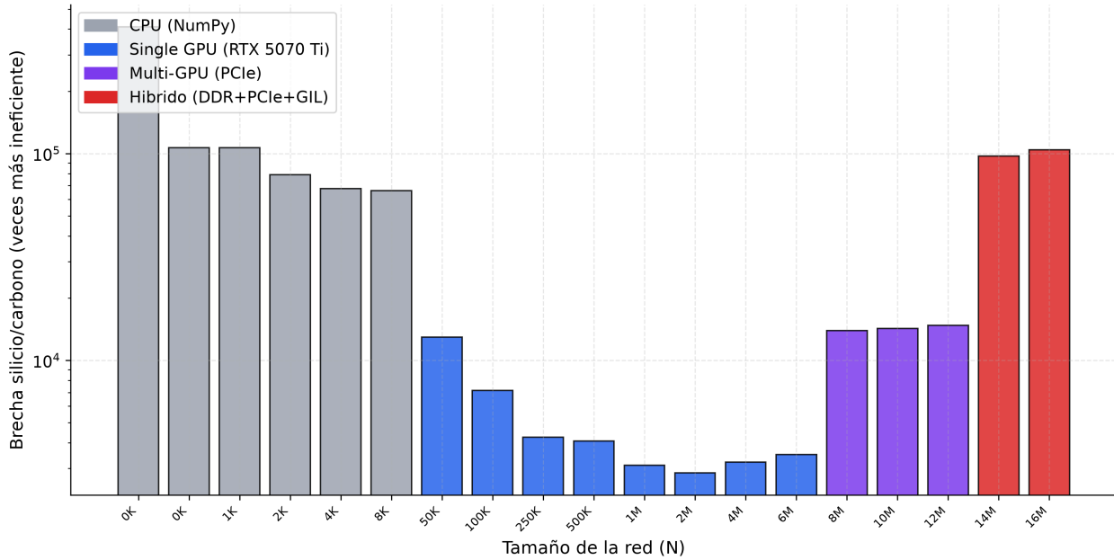
Fig. 5 — La brecha silicio/carbono no es monotonica: es emergente de la arquitectura.
