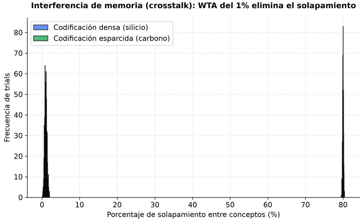
Fig. 3 — Experimento 2: la esparsidad del 1 % reduce el solapamiento conceptual del 80,0 % al 1,03 %.
