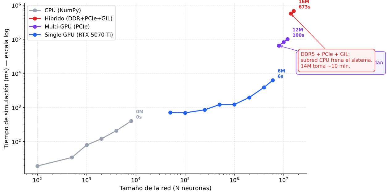
Cuello de botella de Von Neumann hecho visible: tiempo de cómputo por tier de hardware
