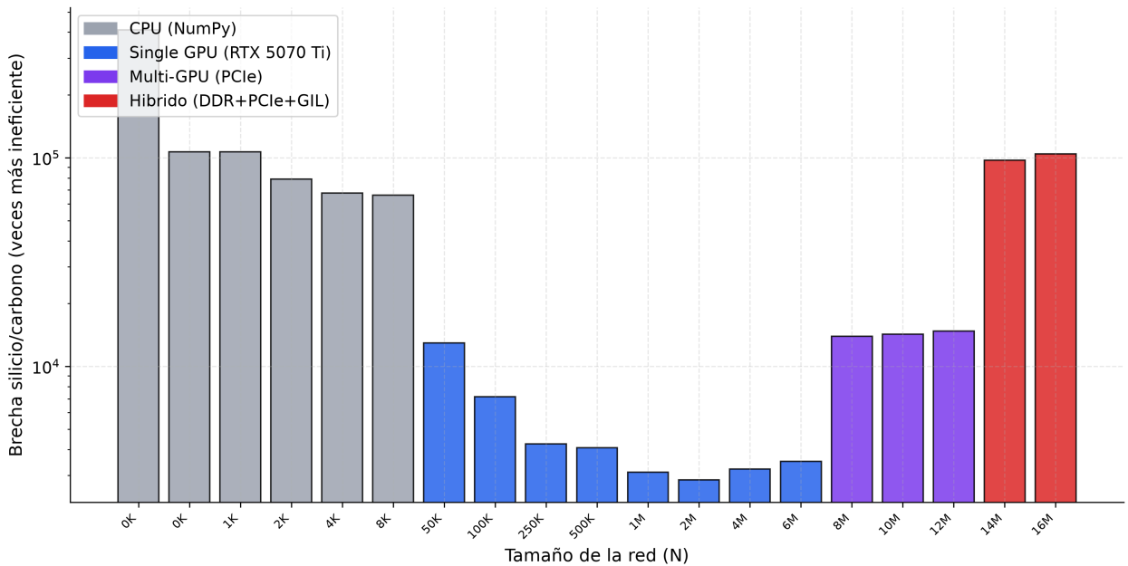
Brecha de eficiencia silicio/carbono por escala y tier
