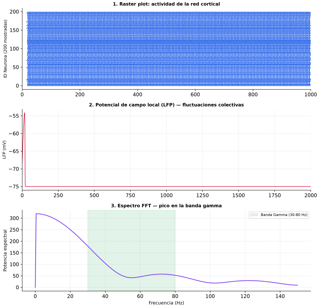
Fig. 6 — Experimento 4: la actividad oscilatoria beta-gamma emerge de la física pasiva del tejido,
