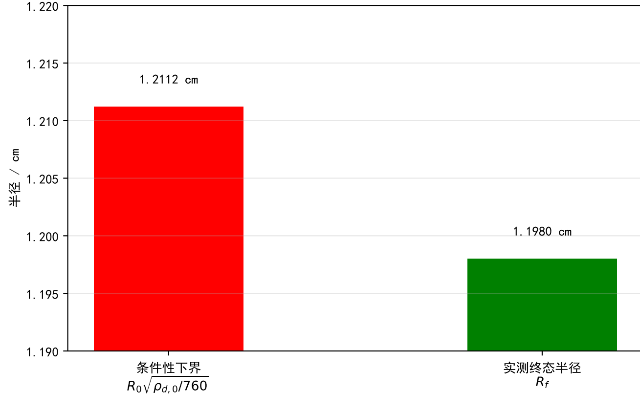
(b) 条件性下界 vs 实测终态半径
