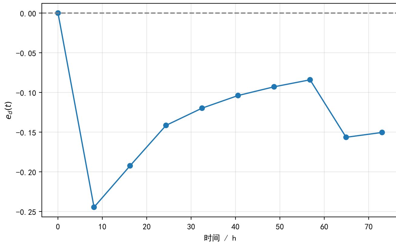
(a) 几何—密度一致性诊断量
