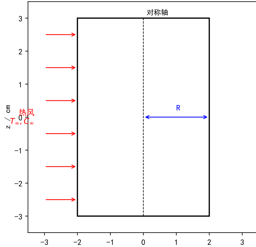
圆柱侧视图与热风边界
