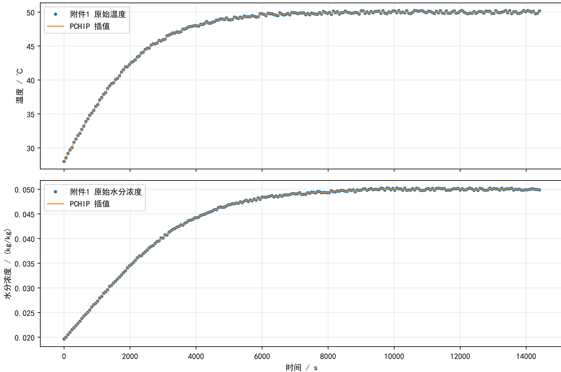
G2 烘房环境数据及插值
