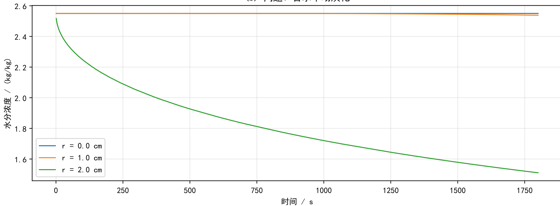
(b) 问题1 含水率场演化
