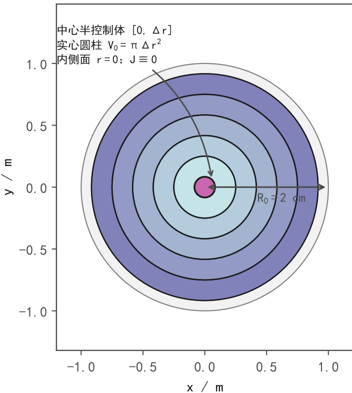
(a) 横截面：环形控制体 + 中心半控制体
