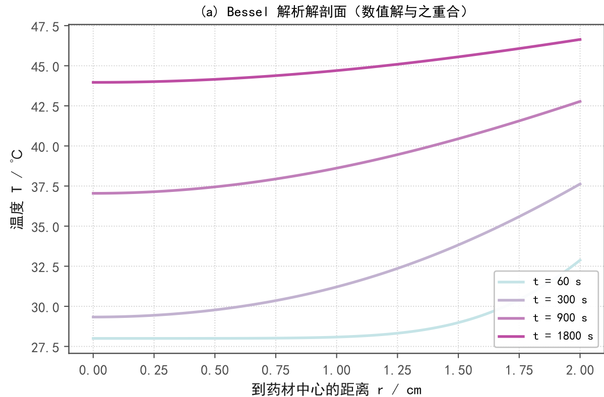
图 FIG-14 解析基准: Bessel 级数与数值解对照 (相对误差 < 0.002%)
