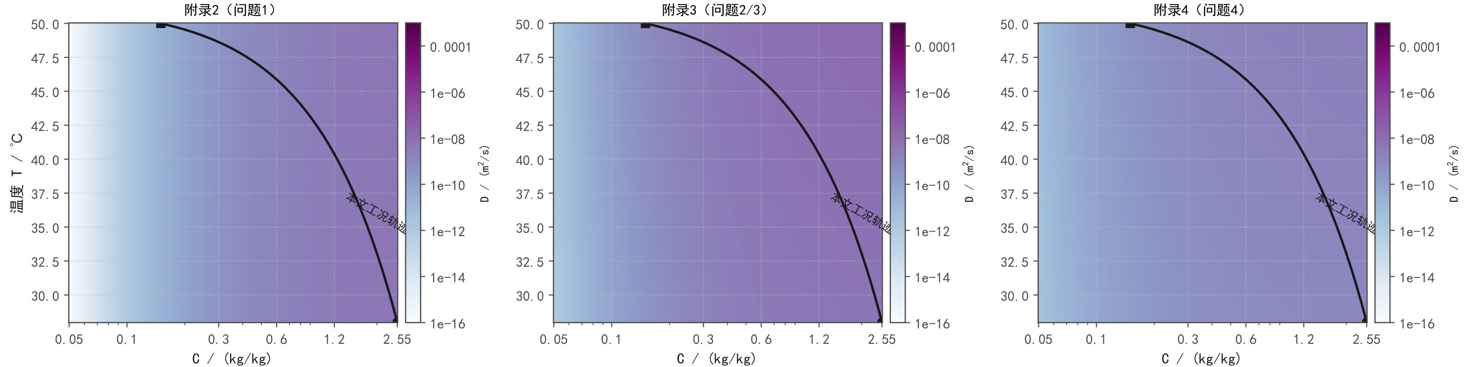
图 FIG-18 附录2/3/4 的扩散系数 D(C, T) 等值线与本文工况轨迹（注意三者的色标范围相同）
