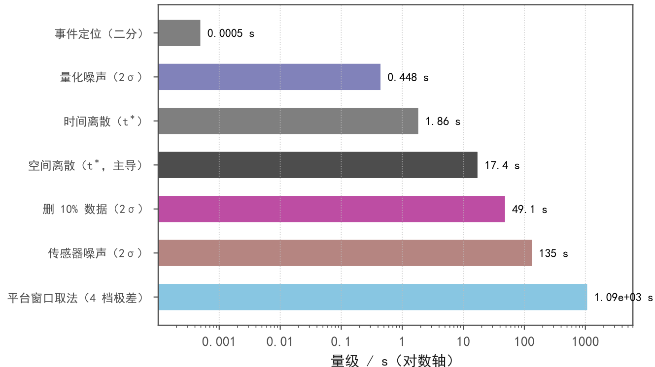
(b) 各项误差/散布的量级对比
