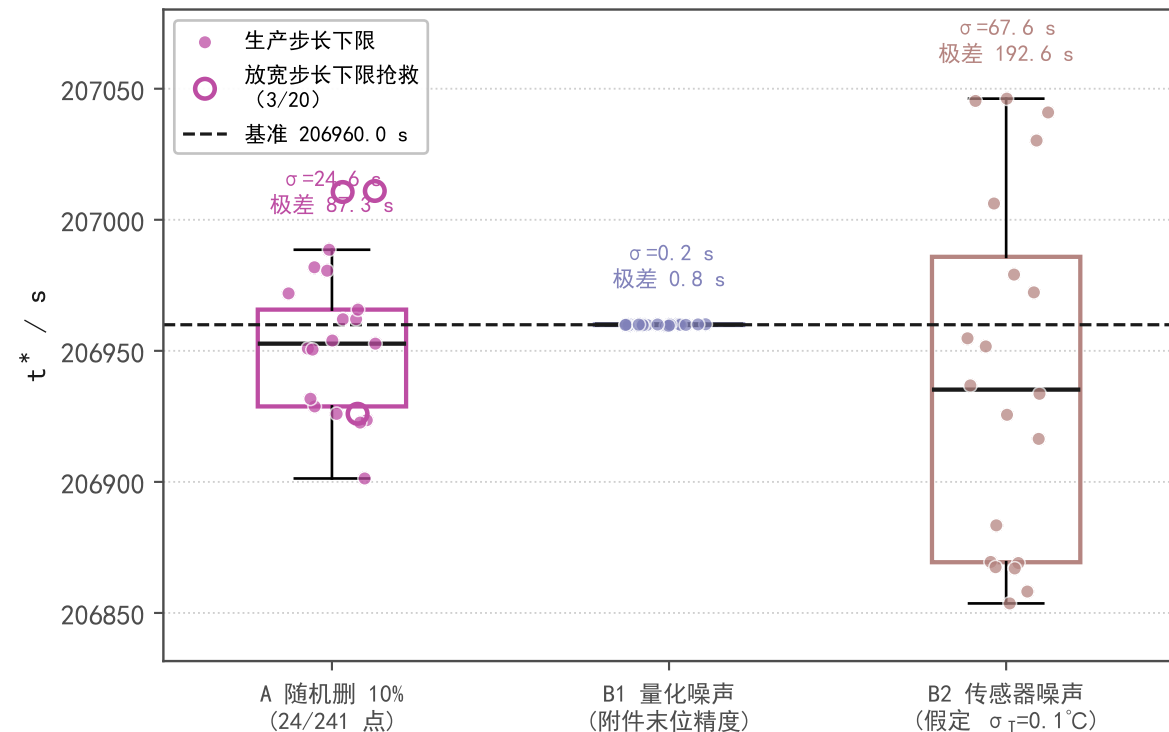
(a) 数据扰动下的 t^* 分布
