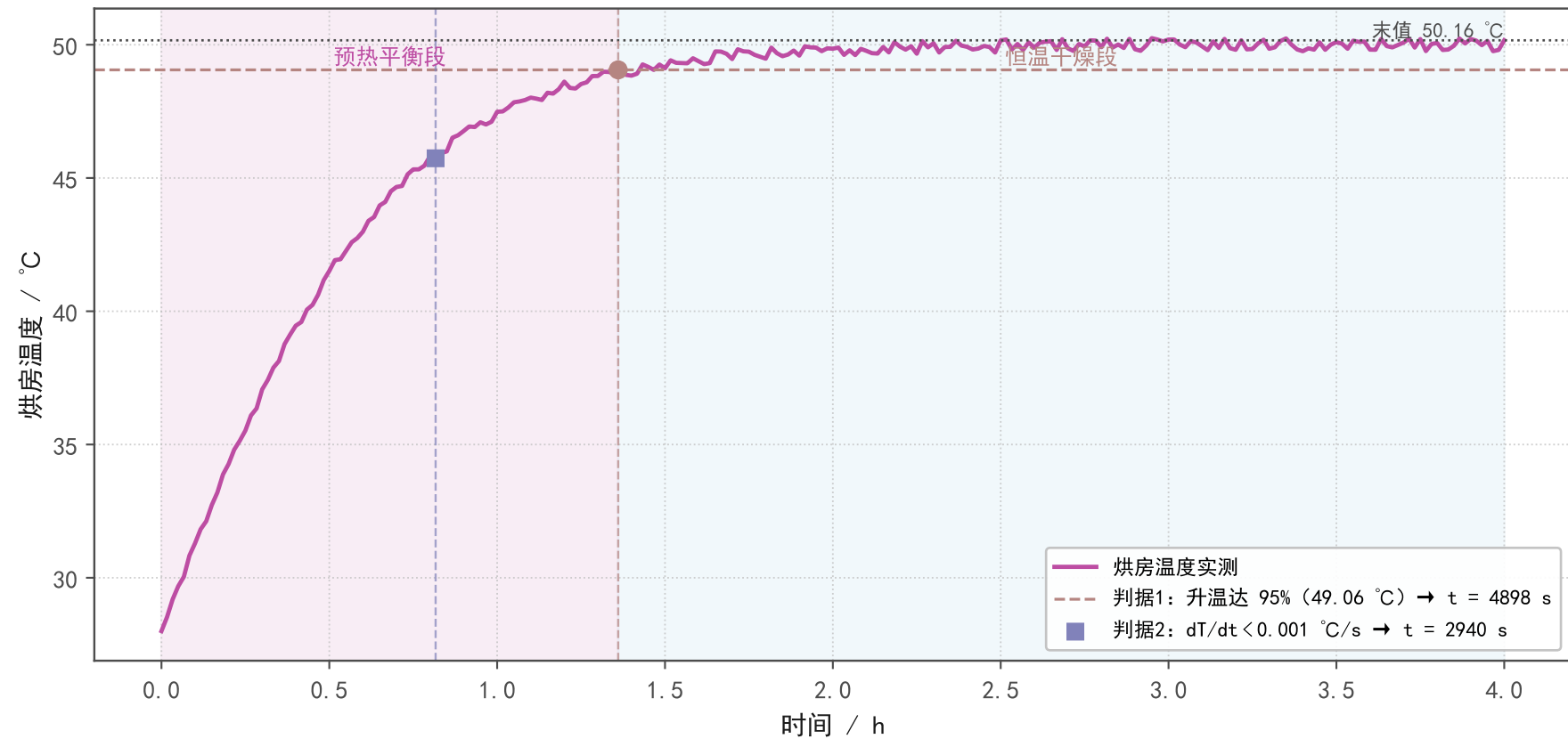
图 G2b 预热/恒温阶段识别
